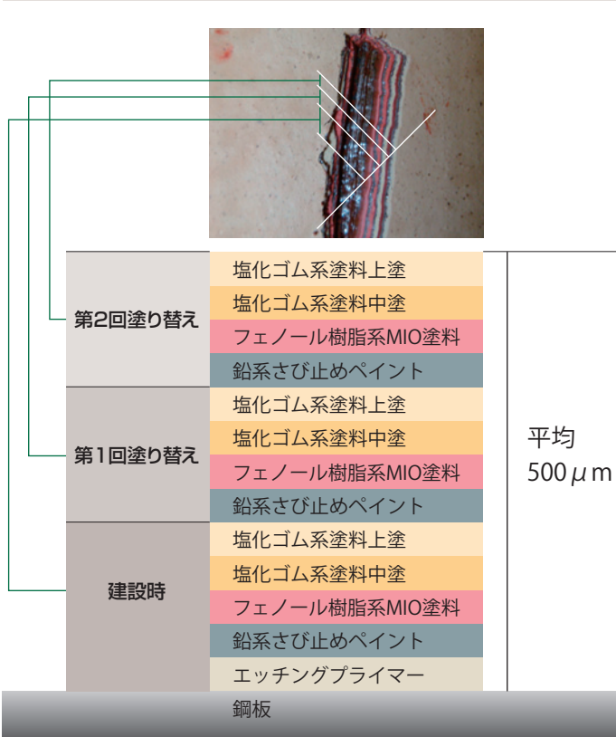
武石高架橋
